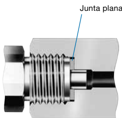
Junta plana
