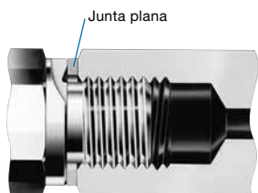
Junta plana
